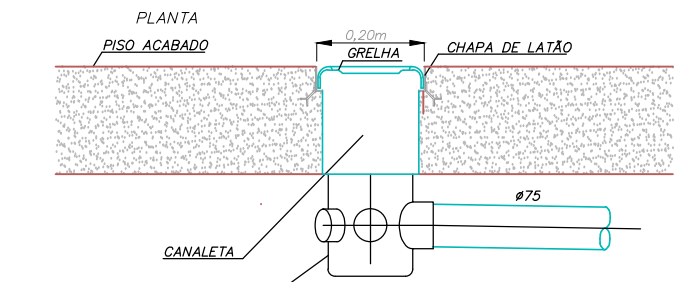
GRELHA DE PISO COM RALO PARA VESTIÁRIOS SEM ESCALA
